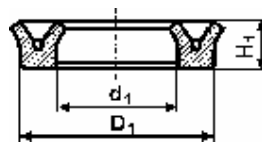
Manžeta Drážková
