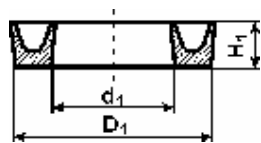
Manžeta U
